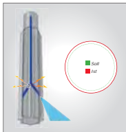
Toleranzfehler durch verstopfte Kühlkanäle
